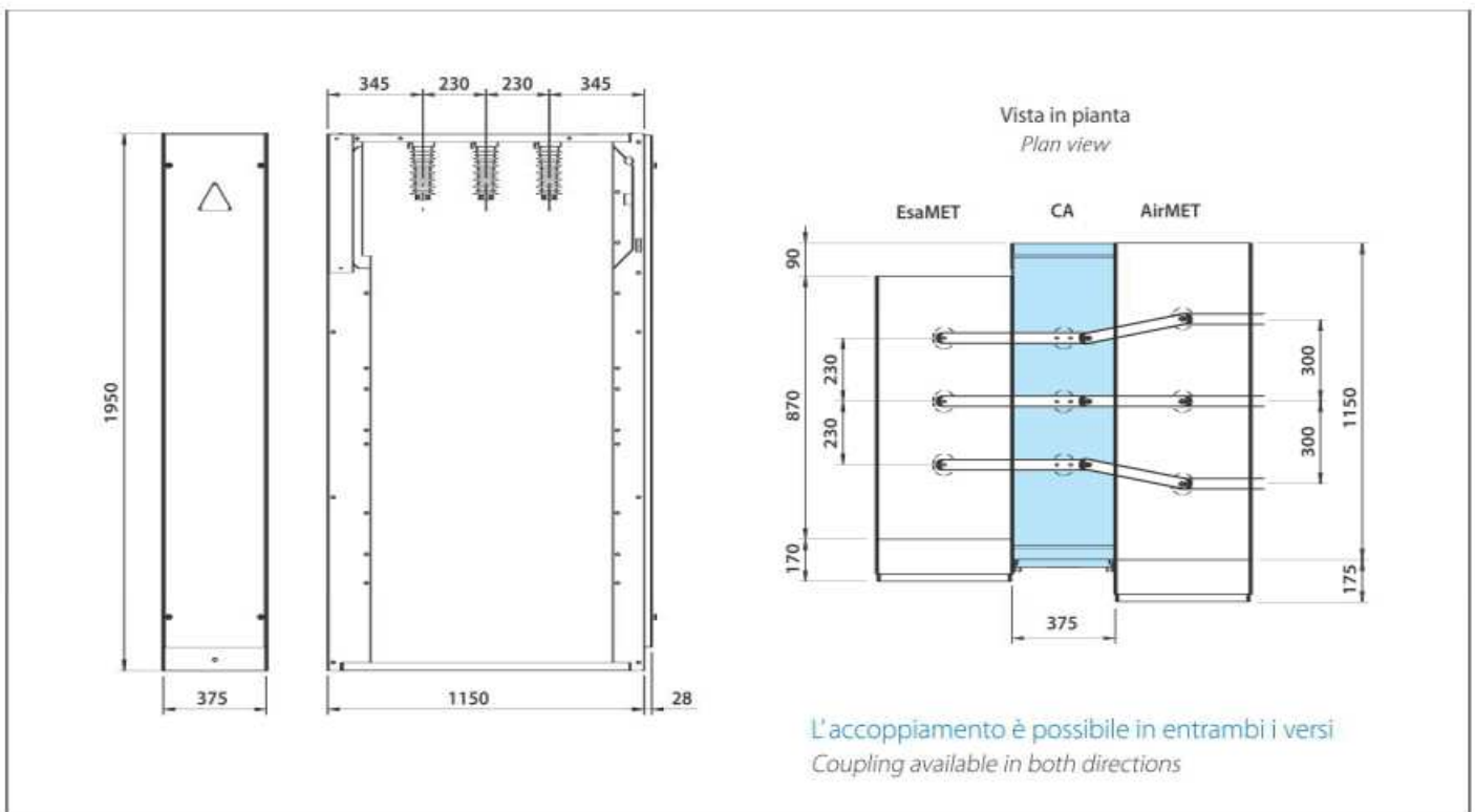
CA - Canala di accoppiamento AirMET- EsaMET AirMET-EsaMET coupling unit
