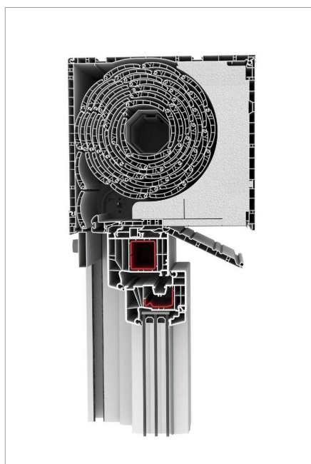
Révision du bas RU permet le plâtrage de l'extérieur et de l'intérieur
