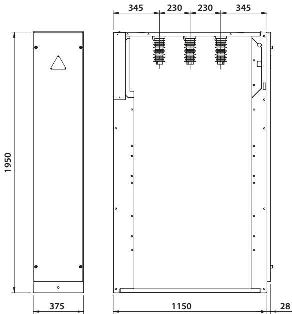
CA - Canala di accoppiamento AirMET- EsaMET AirMET-EsaMET coupling unit
