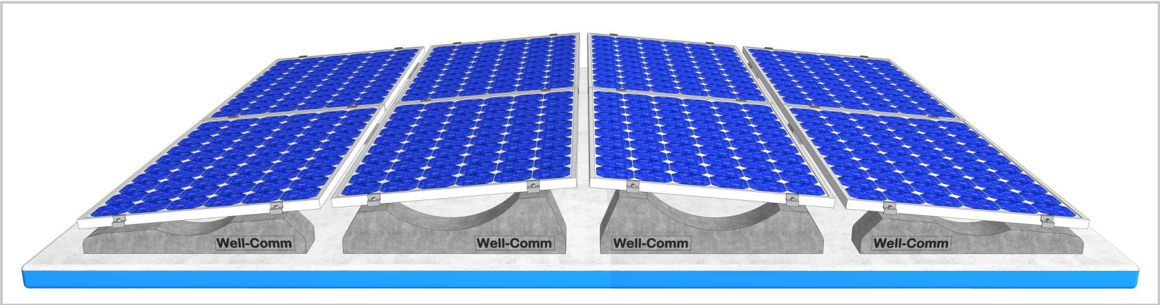
Disposizione Est-Ovest
